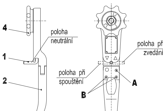
Obr. 6.3 Nastavení délky řetězu
