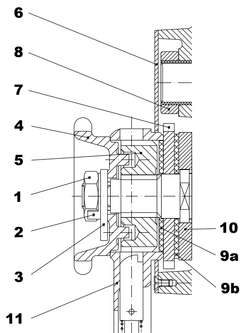
Obr. 11.3 - Montáž brzdy
